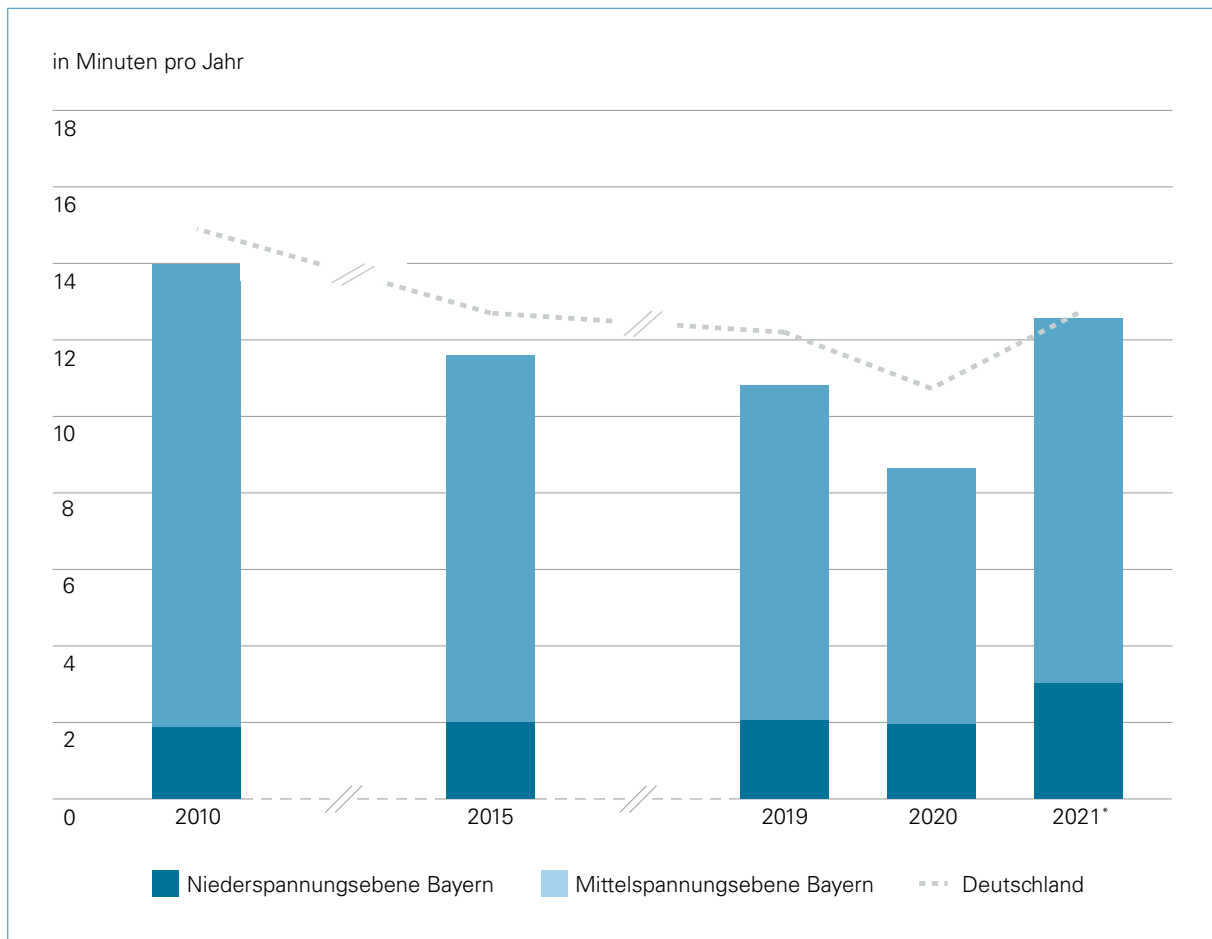
Grafik 2.3 | Entwicklung der durchschnittlichen Stromunterbrechungsdauer je Letztverbraucher nach Netzebene und Jahr in Bayern und bundesweit (Datenbasis: BNetzA)
