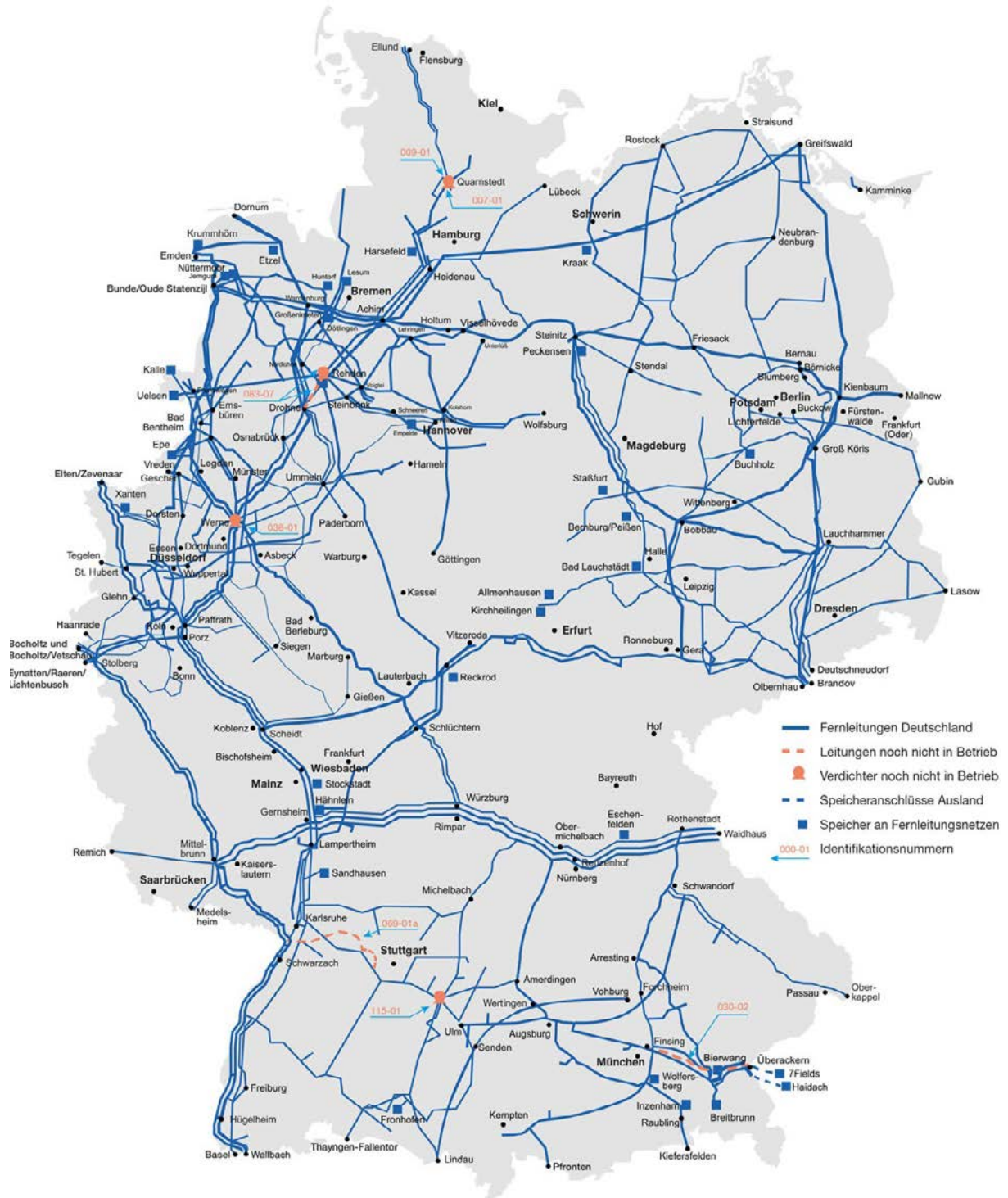
Grafik 2.1 | Startnetz des Netzentwicklungsplans Gas 2020–2030 zum 1. März 2020 (Quelle: Netzentwicklungsplan Gas 2020–2030)
