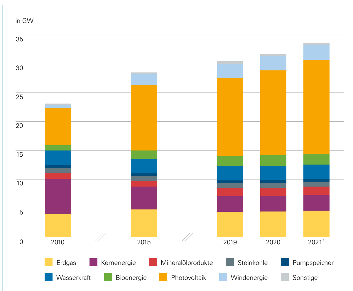
Grafik 2.4 | Entwicklung der installierten Leistung nach Energieträgern in Bayern (Datenbasis: BNetzA, AEE, LfU, LfStat, eigene Erhebungen)
