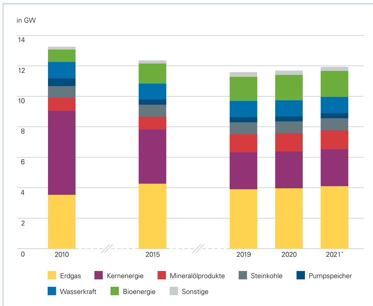
Grafik 2.6 | Entwicklung der gesicherten Erzeugungsleistung 1 in Bayern ohne Netzimportkapazitäten (Datenbasis: BNetzA, AEE, LfU, LfStat, IE Leipzig, eigene Erhebungen)
