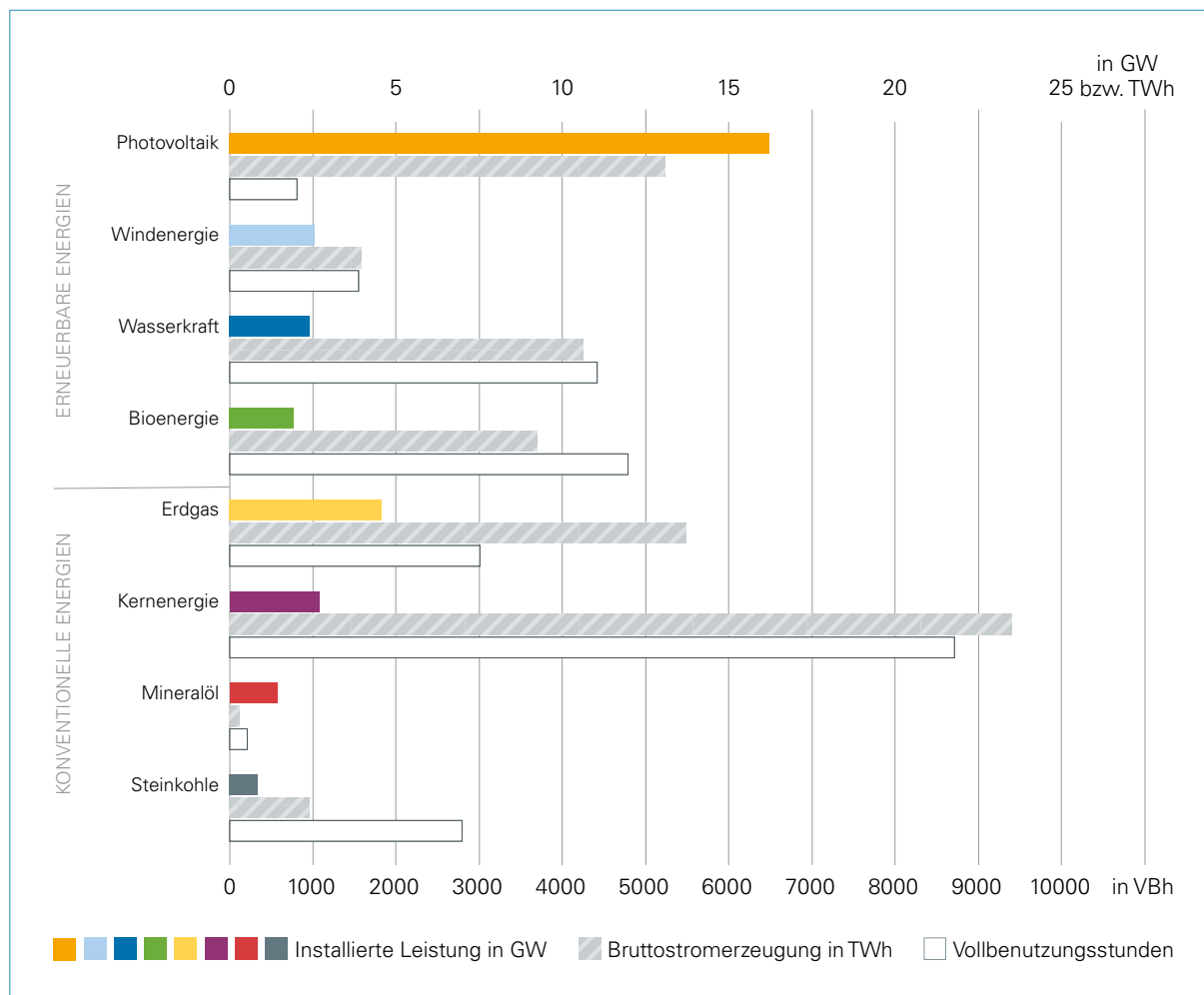
Grafik 2.5 | Installierte Leistung, Bruttostromerzeugung und Vollbenutzungsstunden nach Energieträgern 2021 in Bayern (Datenbasis: BNetzA, AEE, LfU, LfStat, eigene Erhebungen)
